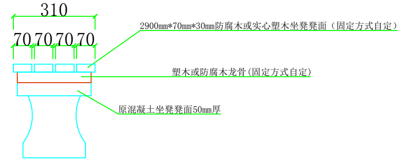
坐凳侧立面图 (mm)
